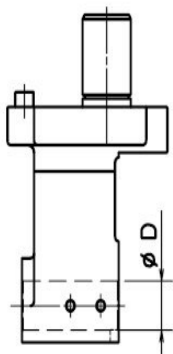
ボーリングバーホルダ ( B ) BORING BAR HOLDER ( B )
