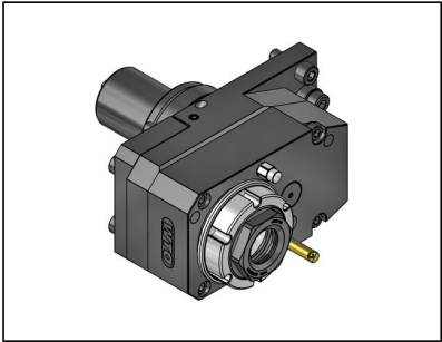
Bohr-Fräseinrichtung - Gerade mit Versatz für Spannzangen DIN 6499B (ER) Externe Kühlmittelzufuhr
